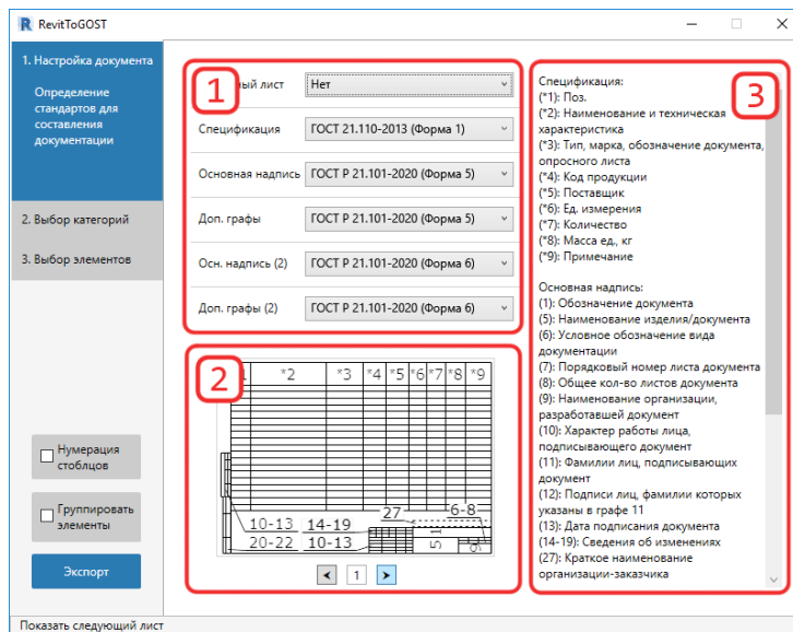
Рис. 3. Вкладка 1 «Определение стандартов для составления документации»
