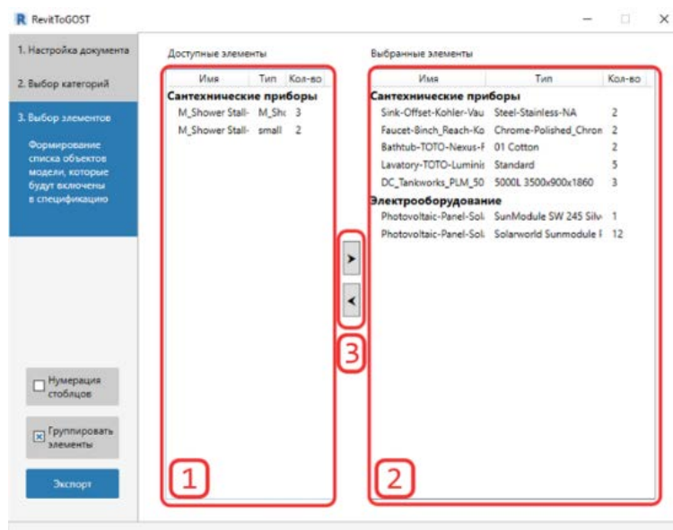
Рис. 5 Вкладка 3 «Выбор элементов»
