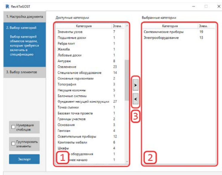
Рис. 4. Вкладка 2 «Выбор категории»
