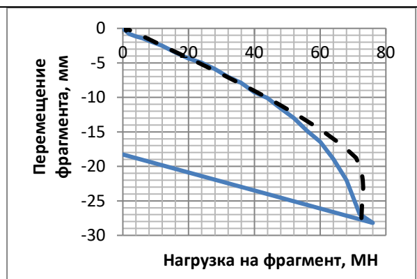
Рис. 20. Характерный результат отладочного моделирования испытания второго этапа сваи 2.
