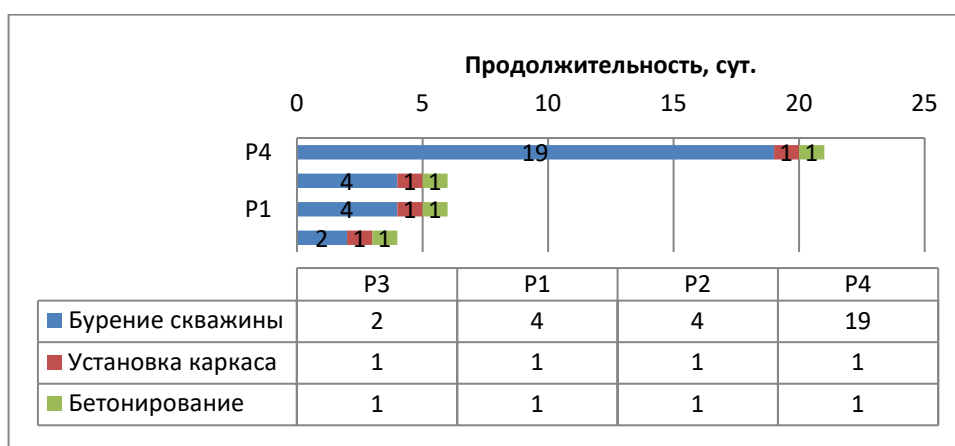
Рис. 8. Распределение времени затраченного на изготовление свай по технологическим процессам.
