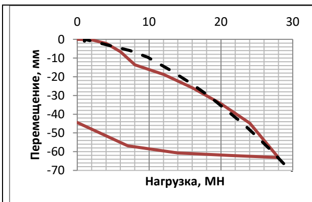
Рис. 19. Характерный результат отладочного моделирования испытания первого этапа сваи 1.
